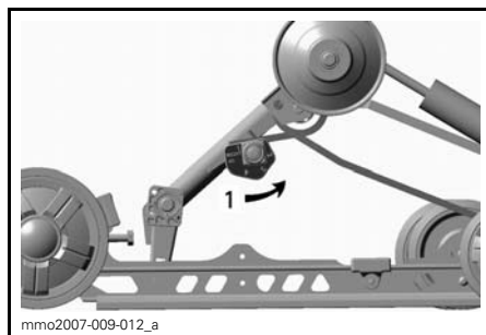
TYPIQUE — SC-5M — CÔTÉ DROIT 1. Régler la précharge du ressort
