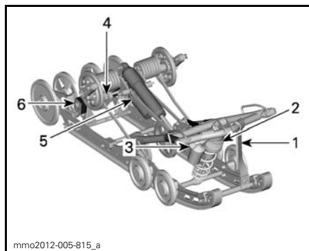
MX Z X-RS - rMOTION - COMPOSANTS RÉGLABLES
