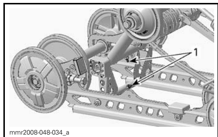
SÉRIES MX Z X MC ET GSX 1. Raccords de graissage
