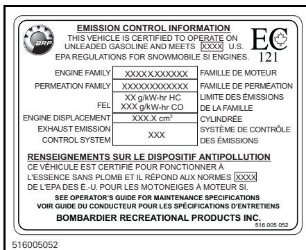
516005052 ÉTIQUETTE DE CONFORMITÉ 1 - DANS LE COMPARTIMENT MOTEUR
