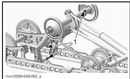
SÉRIES RENEGADE ET GRAND TOURING 1. Raccords de graissage
