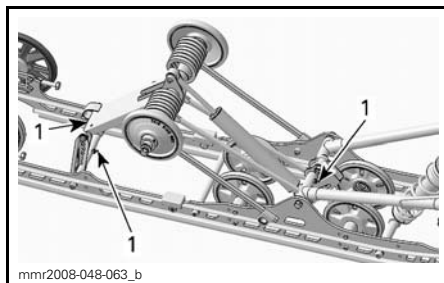
SÉRIE SUMMIT 1. Raccords de graissage
