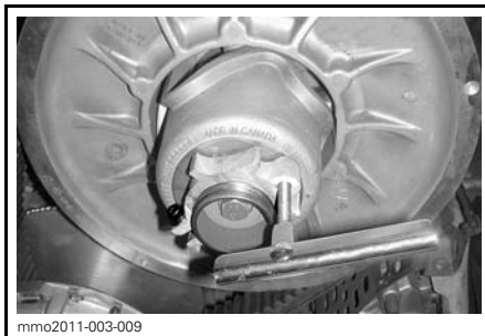
mmo2011-003-009 MANDRIN DE POULIE MENÉE SUR UN DISPOSITIF DE RÉGLAGE EN ALUMINIUM
