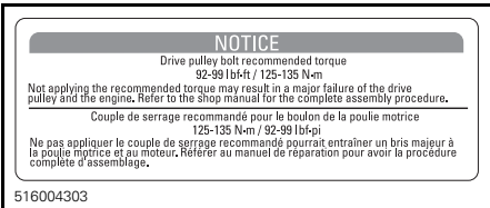
SUR LE GARDE-COURROIE D'ENTRAÎNEMENT
