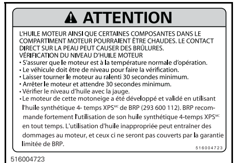
MODÈLE 1200 4-TEC - DANS LE COMPARTIMENT MOTEUR
