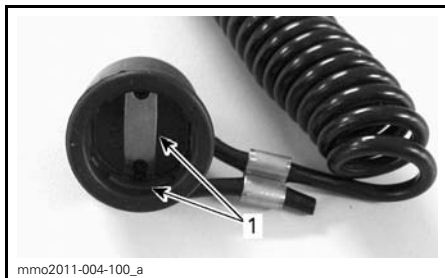
mmo2011-004-100_a CAPUCHON DU CORDON D'ATTACHE
