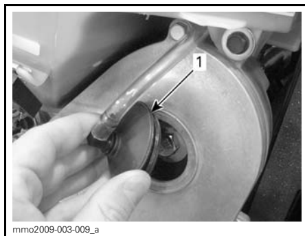
TIPIQUE - DESSUS DU CARTER DE CHAÎNE 1. Bouchon de remplissage
