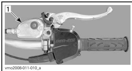
TYPIQUE 1. Réservoir de liquide de frein avant
