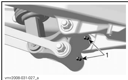
LEVIER COUDÉ 1. Graisseurs
