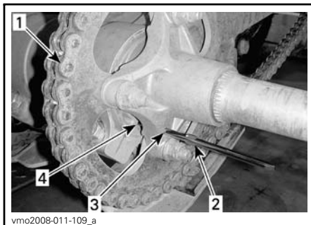
1. Chaîne d'entraînement 2. Lame de tournevis (trousse à outils) 3. Moyeu de roue dentée 4. Carter d'essieu excentrique
