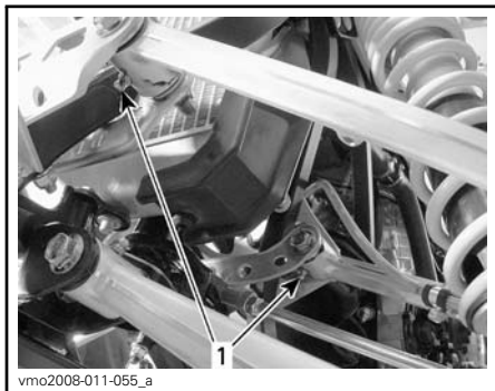
TYPIQUE — BRAS DE SUSPENSION SUPÉRIEUR 1. Graisseurs
