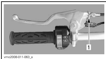
1. Écrou autobloquant
