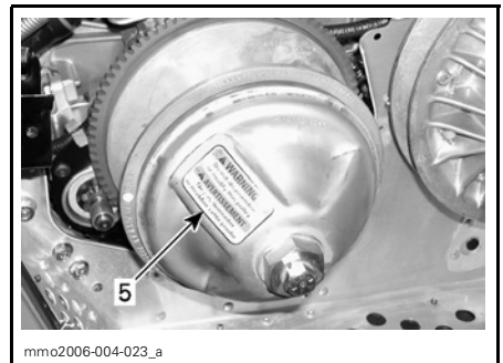
POULIE D'ENTRAÎNEMENT — REFROIDISSEMENT PAR VENTILATEUR
