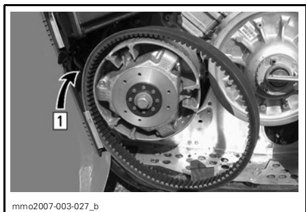
Étape 1: Placer la courroie entre les demi-poulies d'entraînement
