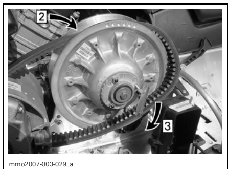
Étape 2: Ensuite, entre les demi-poulies menées
