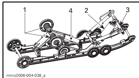
TIPIQUE — SUSPENSION DE SC-136
