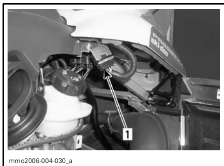
1. Faisceau de fils du capot
