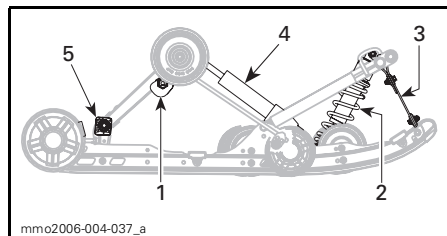
TIPIQUE — SUSPENSION DE SC-4
