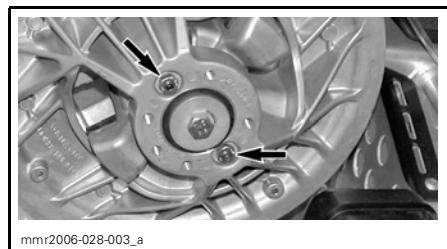
– Desserrer les deux écrous de réglage de la poulie menée.
