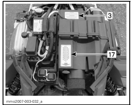
SILENCIEUX D'ADMISSION D'AIR (CÔTÉ MOTEUR) — REFROIDISSEMENT PAR LIQUIDE
