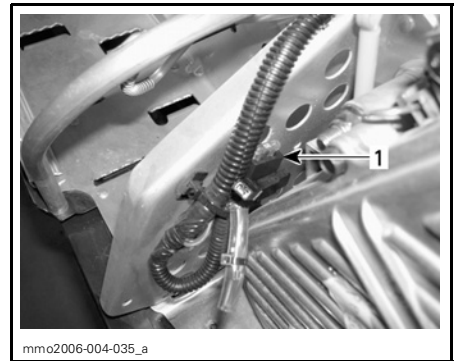
MODÈLES À DÉMARRAGE MANUEL — DERRIÈRE LE REPOSE-PIED DROIT 1. Fusible de protection de masse
