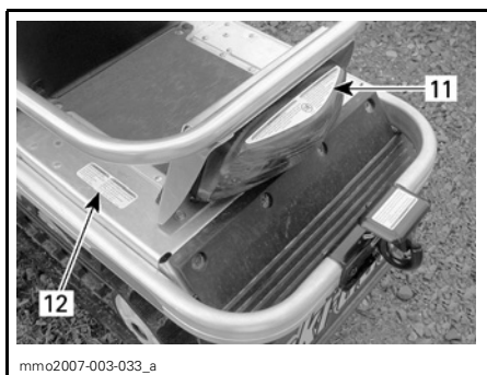
PORTE-BAGAGES ARRIÈRE — TUNDRA/EXPEDITION/LEGEND (DEUX PLACES)
