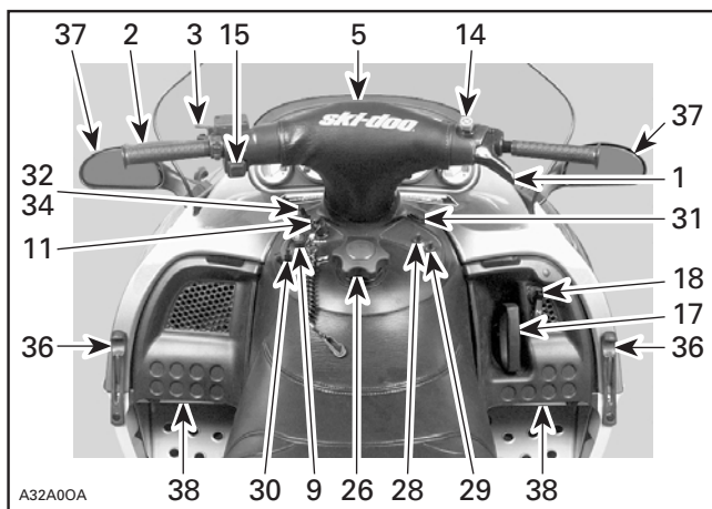
TYPIQUE — MODÈLES À DÉMARREUR ÉLECTRIQUE, REFROIDIS PAR LIQUIDE
