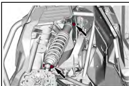
FIXATIONS D'AMORTISSEUR ARRIÈRE
