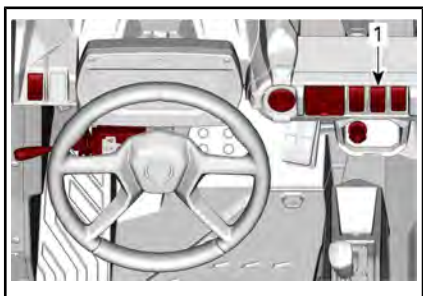
1. Interrupteur de verrouillage du différentiel
