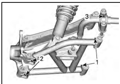
PARTI RIMOSSE PER CHIAREZZA - DISPOSITIVI DI FISSAGGIO AMMORTIZZATORE ANTERIORE
