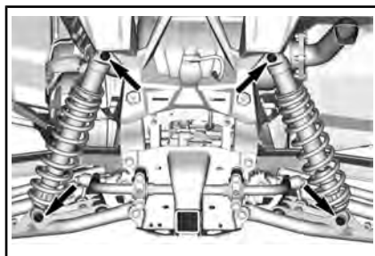
DISPOSITIVI DI FISSAGGIO AMMORTIZZATORE POSTERIORE
