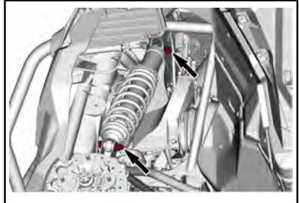
DISPOSITIVI DI FISSAGGIO AMMORTIZZATORE ANTERIORE
