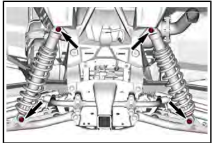
DISPOSITIVI DI FISSAGGIO AMMORTIZZATORE POSTERIORE
