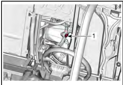
1. Bougie avant
