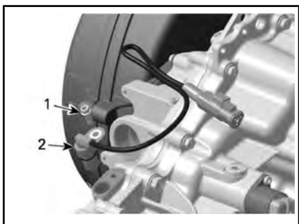
VÁRIAS PEÇAS REMOVIDAS PARA MELHOR VISUALIZAÇÃO
