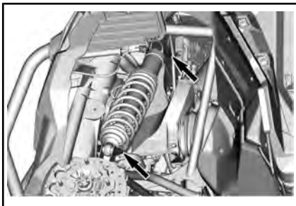
PEÇAS REMOVIDAS PARA MELHOR VISUALIZAÇÃO - FIXADORES DO AMORTECEDOR DIANTEIRO
