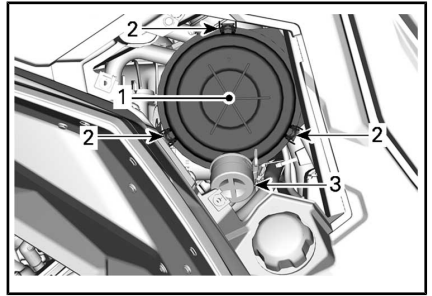
CÔTÉ DROIT DU VÉHICULE, SOUS LA BOÎTE DE CHARGEMENT
