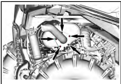
TYPIQUE - ÉCROUS ET BOULONS DE FIXATION DU TUYAU D'ÉCHAPPEMENT ARRIÈRE
