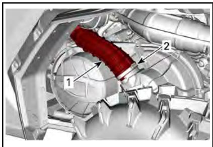
1. CVT-luftinntaksslange 2. Klemme
