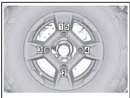
TILTREKKINGSREKKEFØLGE
