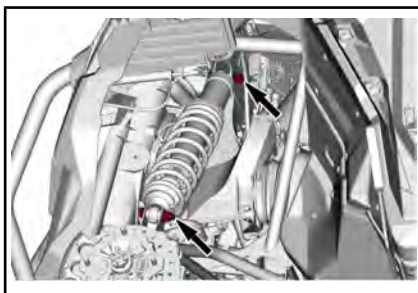
STØTDEMPERFESTER FORAN
