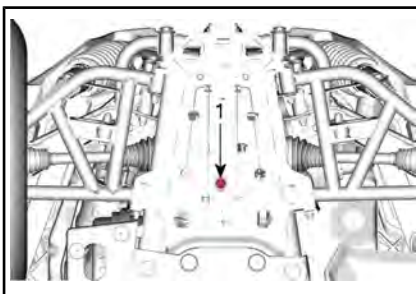
1. Oljedräneringsplugg
