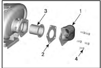
1. Uitlaatpijp 2. Pakking (wegwerp) 3. Vonkafleider 4. Schroef
