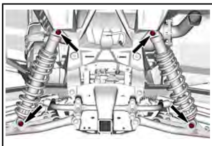
FIXATIONS D'AMORTISSEUR ARRIÈRE
