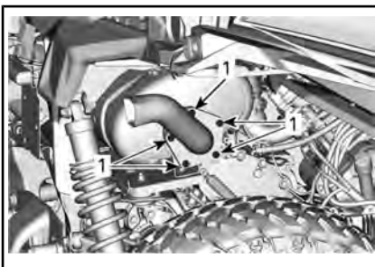
1. Vis de fixation du tuyau arrière
