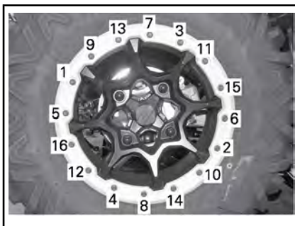
TYPISCH - AANDRAAIVOLGORDE
