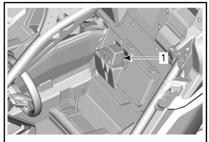
1. Zekeringdoos achter
