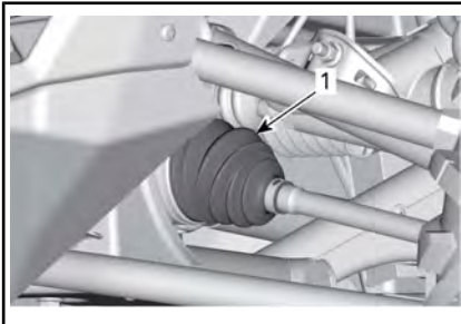
VOORZIJD VOERTUIG
