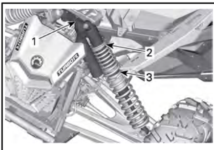
STANDAARD - ZONDER TERUGSLAG-DEMPING - VOORWIELOPHANGING
