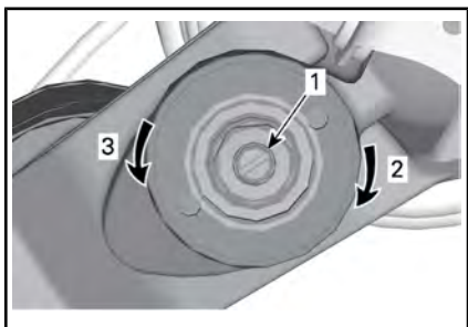
COMPRESSIEDEMPING BIJ LAGE SNELHEID (GEBRUIK EEN SCHROEVENDRAAI-ER)
