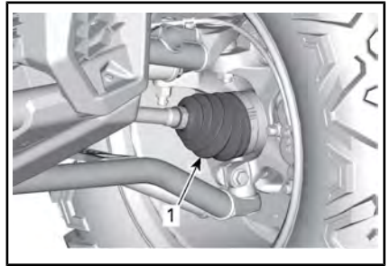
VOORZIJD VOERTUIG
