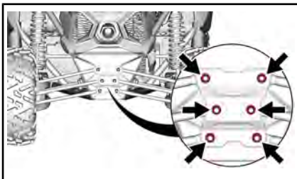
TYPISCH - STABILISATIESTANG VOORAAN
