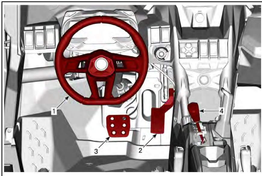
TÍPICO - PIEZAS RETIRADAS PARA MAYOR CLARIDAD
