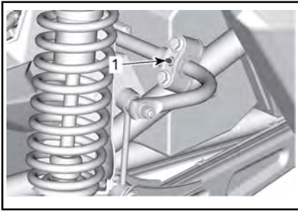
TÍPICO: BARRA ESTABILIZADORA TRASERA
