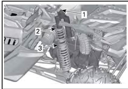
TÍPICO - SIN AMORTIGUACIÓN DE REBOTE - SUSPENSIÓN TRASERA
