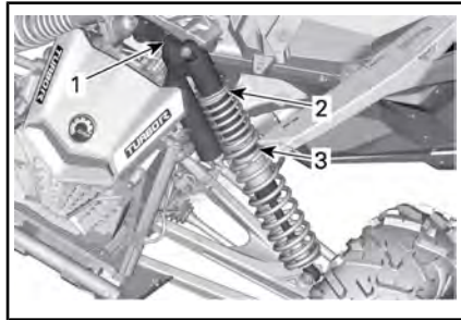
TÍPICO - SIN AMORTIGUACIÓN DE REBOTE - SUSPENSIÓN DELANTERA
