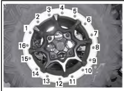
TÍPICO: SECUENCIA DE APRIETE FINAL
