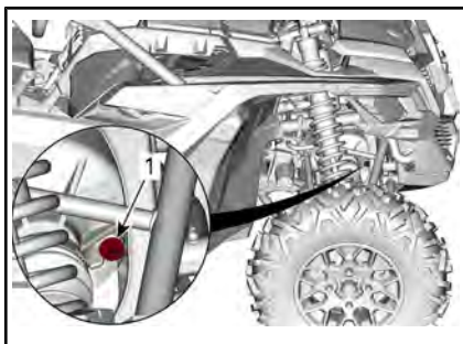
MODELOS EQUIPADOS CON DIFERENCIAL DELANTERO VISCO-LOK
