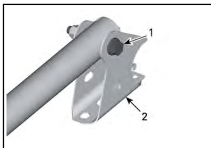
PUNTOS DE ANCLAJE DELANTEROS EN LA POSICIÓN ALTA
