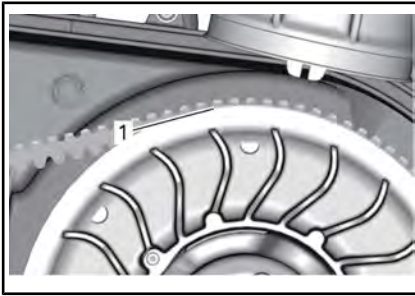
1. Porción más baja de los piñones alineada con el borde de la polea pasiva
