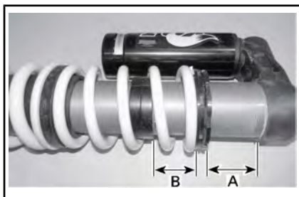
典型示例 - 交叉调整 - 后减震器
