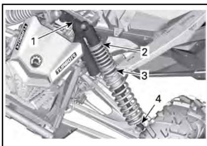
典型示例 - 带回弹阻尼 - 前悬架
