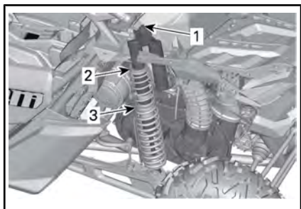
典型示例 - 不带回弹阻尼 - 后悬架
