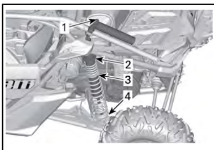
典型示例 - 带回弹阻尼和外置储液罐 - 后悬架
