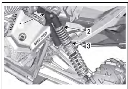
典型示例 - 不带回弹阻尼 - 前悬架
