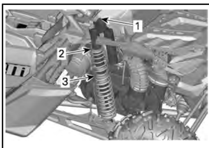
TYPIQUE - SUSPENSION ARRIÈRE
