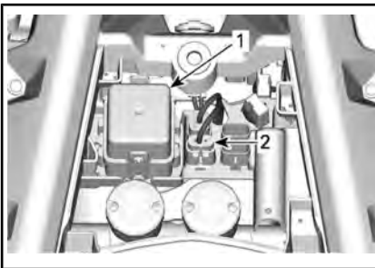
1. Boîte à fusibles avant 2. Fusible DPS
