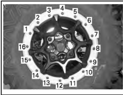
TYPIQUE - SÉQUENCE DE SERRAGE FINAL
