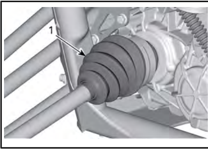
ЗАДНЯЯ ЧАСТЬ МОТОВЕЗДЕХОДА (КОМПОНЕНТЫ СНЯТЫ ДЛЯ НАГЛЯДНОСТИ)
