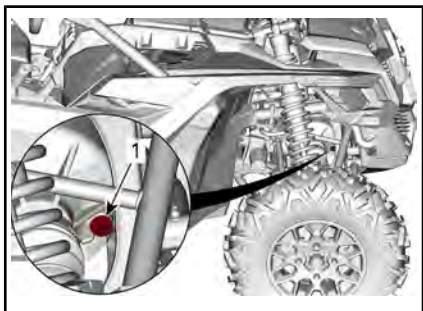
МОДЕЛИ С ПЕРЕДНИМ ДИФФЕРЕНЦИАЛОМ Visco-Lok
