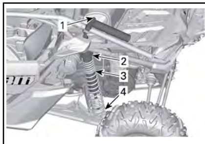
ТИПОВОЙ ВАРИАНТ - С ДЕМПФИРОВАНИЕМ ХОДА ОТБОЯ И ВЫНОСНЫМ РЕЗЕРВУАРОМ - ПЕРЕДНЯЯ ПОДВЕСКА
