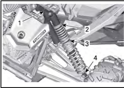
ESEMPIO TIPO - CON SMORZAMENTO IN ESTENSIONE - SOSPENSIONE ANTERIORE
