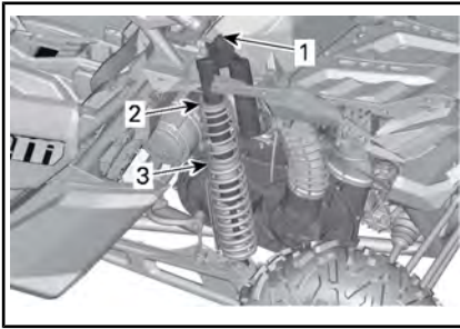
ESEMPIO TIPO - SENZA SMORZAMENTO IN ESTENSIONE - SOSPENSIONE POSTERIORE
