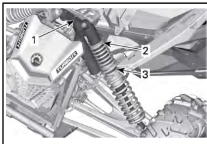
ESEMPIO TIPO - SENZA SMORZAMENTO IN ESTENSIONE - SOSPENSIONE ANTERIORE
