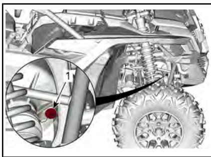
MODELLI DOTATI DI DIFFERENZIALE ANTERIORE VISCO-LOK
