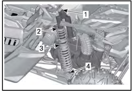
ESEMPIO TIPO - CON SMORZAMENTO IN ESTENSIONE - SOSPENSIONE POSTERIORE
