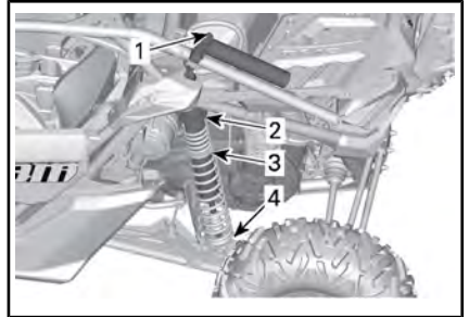
ESEMPIO TIPO - CON SMORZAMENTO IN ESTENSIONE E SERBATOIO REMOTO - SOSPENSIONE POSTERIORE
