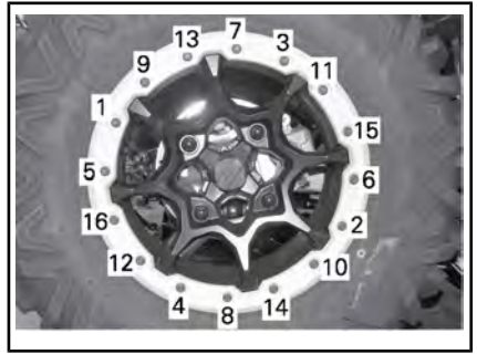
TÍPICO: SECUENCIA DE APRIETE
