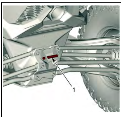
1. Gancho de recuperación trasero
