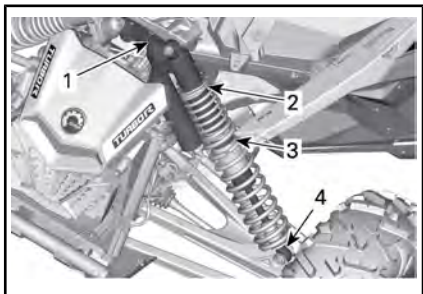
TÍPICO - CON AMORTIGUACIÓN DE REBOTE - SUSPENSIÓN DELANTERA
