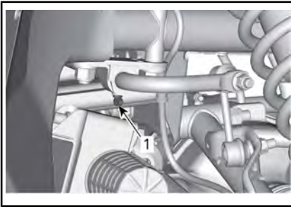
TÍPICA - BARRA ESTABILIZADORA DE LANTERA
