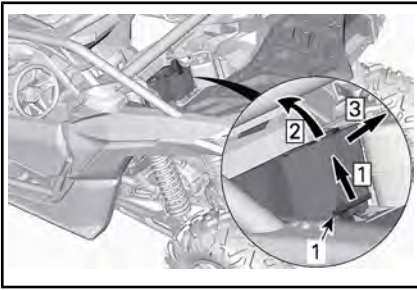
1. Filtro de aire de la CVT
