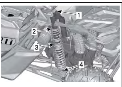
TÍPICO - CON AMORTIGUACIÓN DE REBOTE - SUSPENSIÓN TRASERA
