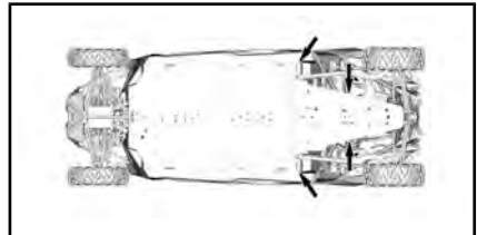
POSICIONES DEL SOPORTE DEL GATO - PARTE TRASERA DEL VEHÍCULO
