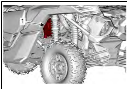
PARTE TRASERA IZQUIERDA DEL VEHÍCULO
