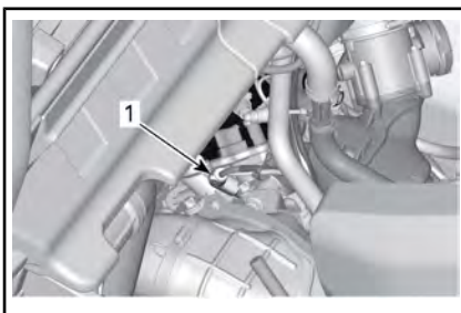
VOORSTE CILINDER (AAN LINKERKANT)
