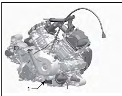
STANDARD - ETICHETTA DEL NUMERO DI SERIE DEL MOTORE
