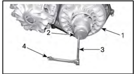
SEQUENZA DI SERRAGGIO DELLA CARENATURA DELLA CVT
