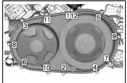
SECUENCIA DE APRIETE DE LA TAPA DE LA CVT (HD8)
