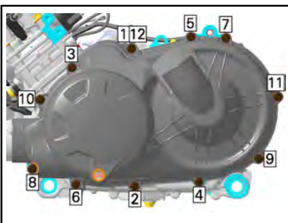
HD5 - ANZUGSREIHENFOLGE DER CVT ABDECKUNG
