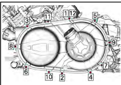
HD10 CVT-ABDECKUNG-ANZUGSREIHENFOLGE
