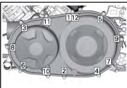
HD8 CVT-ABDECKUNG-ANZUGSREIHENFOLGE
