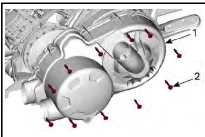
HD5 - ANZUGSREIHENFOLGE DER CVT ABDECKUNG
