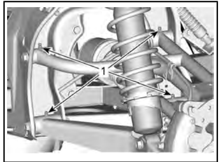
1. Smörjnipplar på bakre bärmarna
