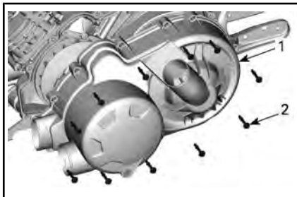
1. Couvercle de la boîte de vitesses CVT 2. Vis du couvercle de la boîte de vitesses CVT
