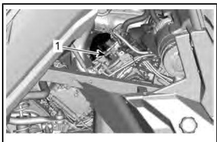
HD8 ET HD10 — CYLINDRE ARRIÈRE (SUR LE CÔTÉ DROIT)
