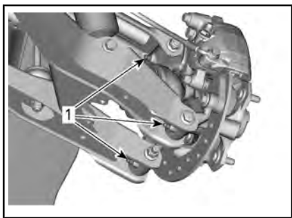
1. Raccords de graissage de fusée arrière
