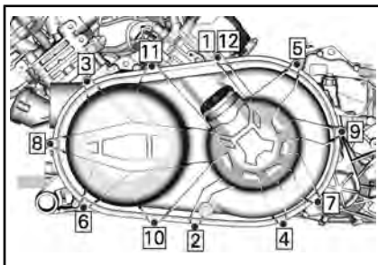
SÉQUENCE DE SERRAGE DU COUVERCLE DE LA BOÎTE CVT HD10
