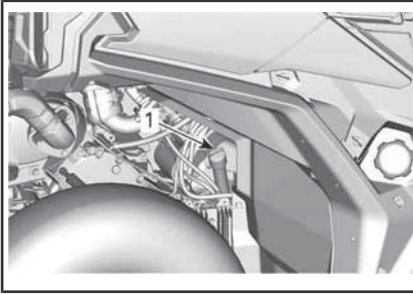
1. Mätsticka för motorolja
