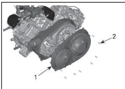
1. CVT-kåpa 2. CVT-kåpskruvar
