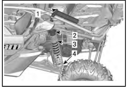
TYPEXEMPEL – MAVERICK X rs OCH X rc TURBO R-MODELLER – BAKFJÄDRING
