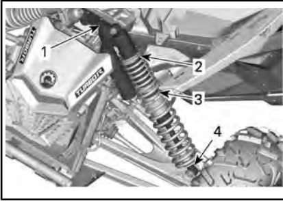
TYPEXEMPEL – MAVERICK X ds-, X rs- OCH XRC TURBO R-MODELLER – FRAMFJÄDRING
