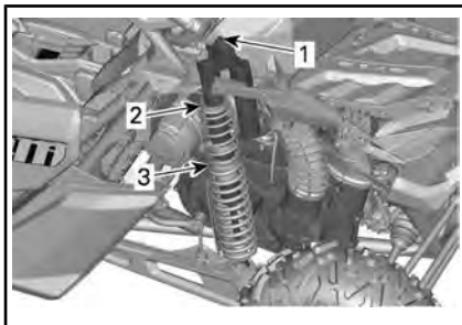
TYPEXEMPEL – MAVERICK TURBO OCH X rc TURBO-MODELLER – BAKFJÄDRING
