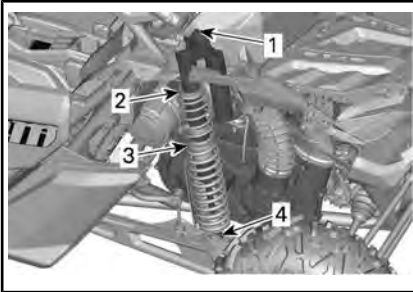
TYPEXEMPEL – MAVERICK X ds-MODELLER – BAKFJÄDRING
