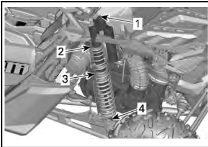
TÍPICO - MODELOS MAVERICK X ds - SUSPENSÃO TRASEIRA
