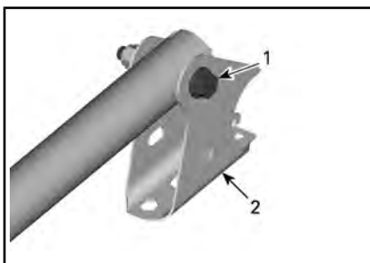
PONTOS DE FIXAÇÃO DIANTEIROS NA POSIÇÃO ALTA
