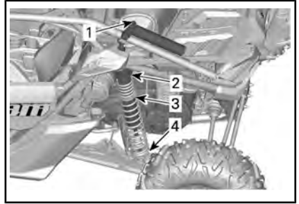
TÍPICO - MODELOS MAVERICK X rsE Xrc TURBO R - SUSPENSÃO TRASEIRA
