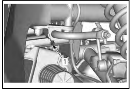
TÍPICO - BARRA ESTABILIZADORA DIANTEIRA
