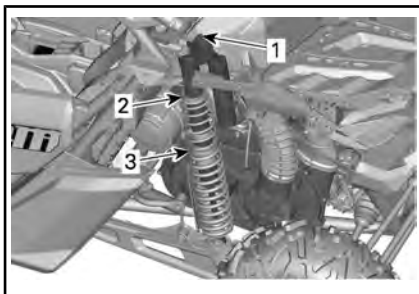
TÍPICO - MODELOS MAVERICK TURBO E X rc TURBO - SUSPENSÃO TRASEIRA
