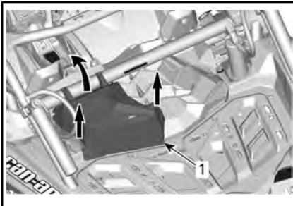
1. Tampa de manutenção
