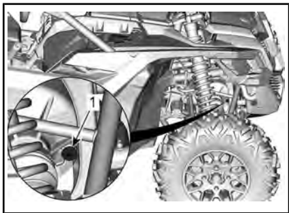
MODELLEN UITGERUST MET VISCO-LOK VOORDIFFERENTIEEL
