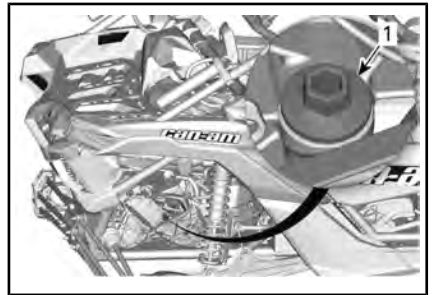
MODELLEN UITGERUST MET VISCO-LOK VOORDIFFERENTIEEL
