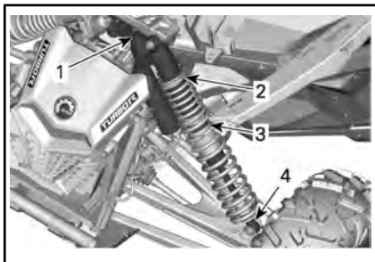
TYPISCH - MAVERICK X ds, X rs EN XRC TURBO R MODELLEN - OPHANGING VOOR
