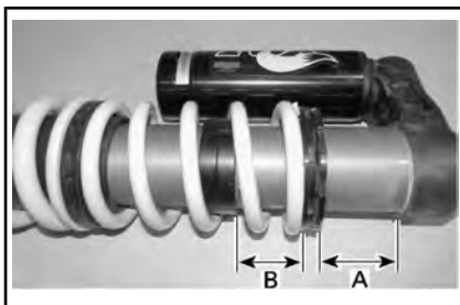
TYPISCH - BIJSTELLING CROSSOVER - ACHTERSCHOKDEMPER
