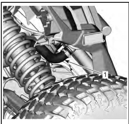
1. Onderste slang
