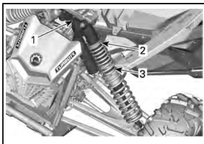
TYPISCH - MAVERICK TURBO EN X rc TURBO MODELLEN - OPHANGING VOOR
