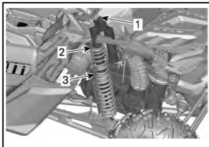
TYPISCH - MAVERICK TURBO EN X rc TURBO MODELLEN - OPHANGING ACHTER
