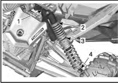
TYPIQUE - MODÈLES MAVERICK X ds, X rs ET X rc TURBO R - SUSPENSION AVANT
