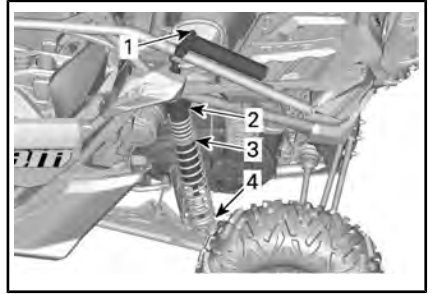
TYPIQUE - MODÈLES MAVERICK X rs ET X rc TURBO R - SUSPENSION ARRIÈRE
