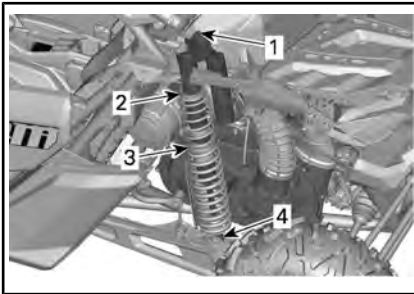
TYPIQUE - MODÈLES MAVERICK X ds - SUSPENSION ARRIÈRE
