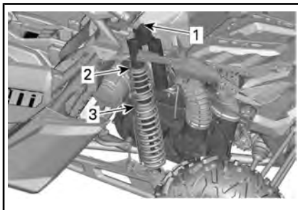
TYPIQUE - MODÈLES MAVERICK TURBO ET X rc TURBO - SUSPENSION ARRIÈRE
