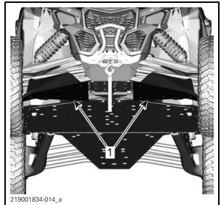
1. A-arm Protector
