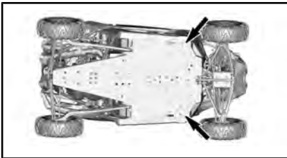
WAGENHEBERSTÜTZBOCK - FAHRZEUGFRONT
