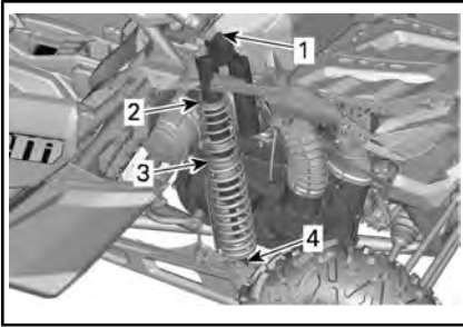
TYPISCH - MAVERICK X ds-MODELLE - HINTERE AUFHÄNGUNG
