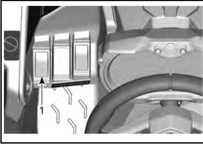
1. Windenschalter
