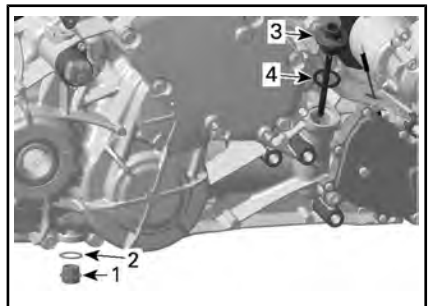
1. Magnetische Ablassschraube 2. Dichtungsring (entsorgen Sie ihn) 3. Schraube für den Getriebeölstand (Messstab) 4. O-Ring
