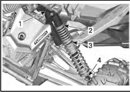
TYPISCH - MAVERICK X ds-, X- rs UND XRC TURBO R-MODELLE - VORDERE AUFHÄNGUNG
