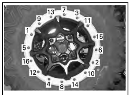
TYPISCH – ANZIEHREIHENFOLGE
