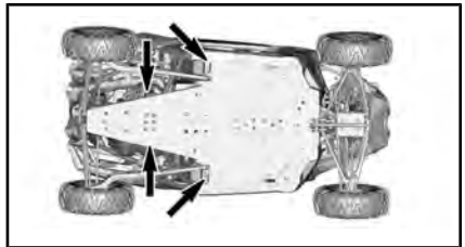
WAGENHEBERSTÜTZBOCK - FAHRZEUGHECK
