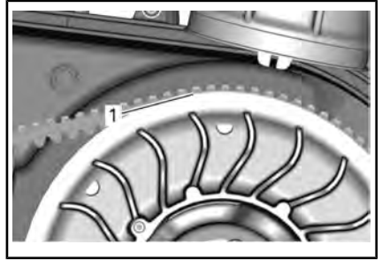
1. Unterster Teil der Zahnräder bündig mit der Außenfläche des Antriebsriemens
