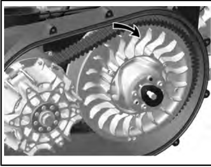
1. Unterster Teil der Zahnräder bündig mit der Außenfläche des Antriebsriemens
