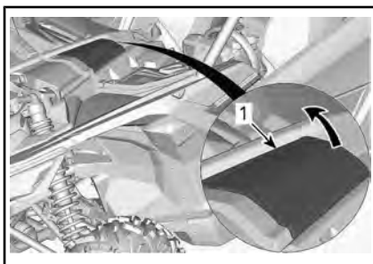
1. Vorderer Wartungsabdeckung
