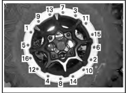
TYPISCH - AANDRAAIVOLGORDE
