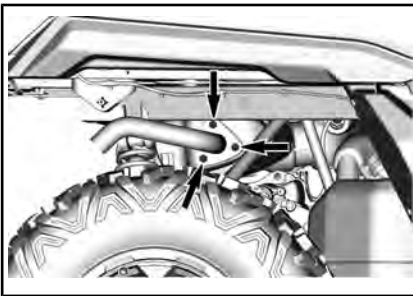
VIS DE FIXATION DU TUYAU ARRIÈRE
