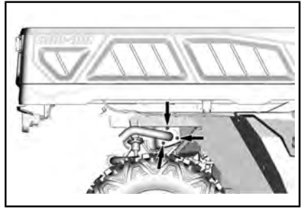
VIS DE FIXATION DU TUYAU ARRIÈRE
