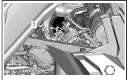
HD10 — VÉRIN ARRIÈRE (SUR LE CÔTÉ DROIT)
