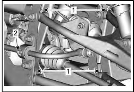
SOSPENSIONE ANTERIORE - SITUAZIONE TIPICA
