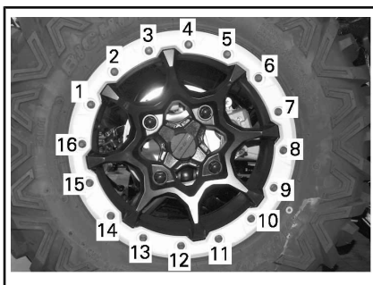
TYPIQUE - SÉQUENCE DE SERRAGE FINALE
