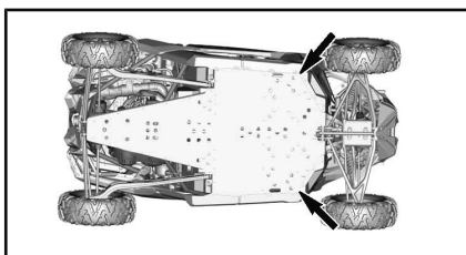
POSITIONS DES CHANDELLES - AVANT DU VÉHICULE
