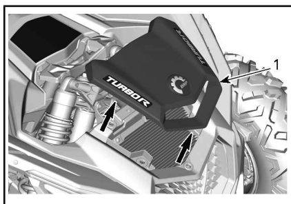
TYPIQUE - COUVERCLE DE CARÉNAGE
