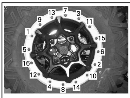
TYPIQUE - SÉQUENCE DE SERRAGE
