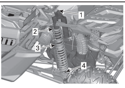
TÍPICO - MODELOS MAVERICK MAX X dsDS - SUSPENSIÓN TRASERA
