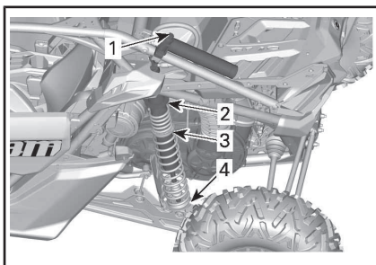
TÍPICO - MODELOS MAVERICK MAX X rsRS - SUSPENSIÓN TRASERA
