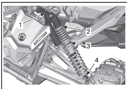
TÍPICO - MODELOS MAVERICK MAX X dsDS Y XrsRS - SUSPENSIÓN DELANTERA
