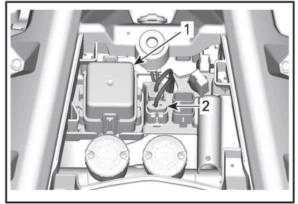
1. Caja de fusibles delantera 2. Fusible de la DPS
