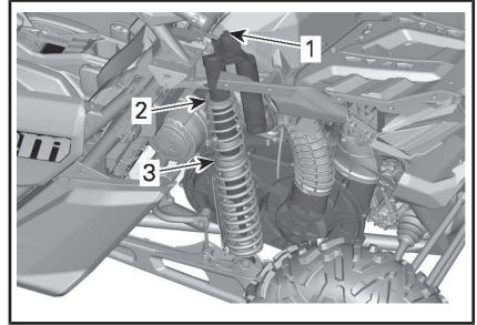
TÍPICO - MODELOS MAVERICK MAX - SUSPENSIÓN TRASERA
