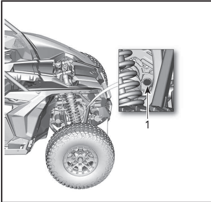
MODELOS EQUIPADOS CON DIFERENCIAL DELANTERO SMART-LOK
