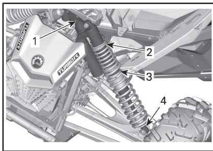
典型示例 - Maverick MAX x ds 和 x rs 车型 - 前悬架
