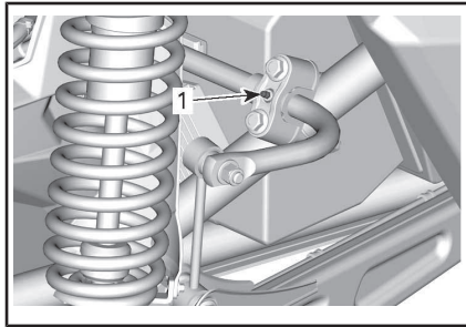
典型示例 - 后平衡杆
