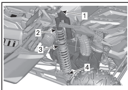
典型示例 - MAVERICK MAX X DS 型号 - 后悬架
