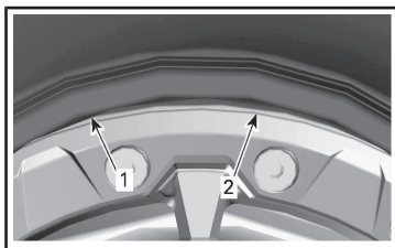
典型示例 轮胎外胎圈 防脱圈内环凸肩
