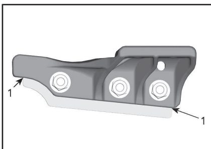
1. 磨损极限
