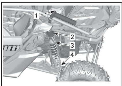
典型示例 - Maverick MAX X rs 车型 - 后悬架
