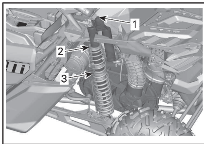
典型示例 - Maverick MAX 车型 - 后悬架
