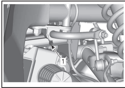
典型示例 - 前平衡杆
