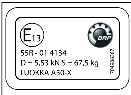
VETOKOUKUSSA
