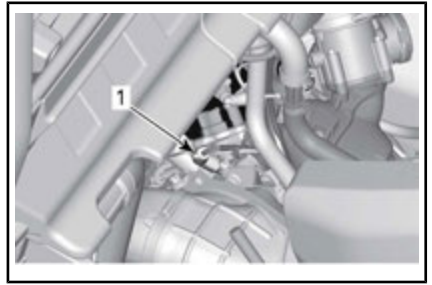
LADO IZQUIERDO — CILINDRO DELANTERO (DEL LADO IZQUIERDO)
