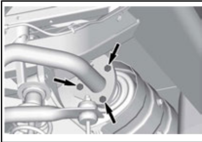
PERNOS DE FIJACIÓN DEL TUBO DE ESCAPE
