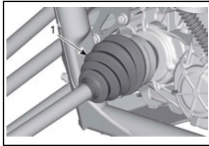
ARRIÈRE DU VÉHICULE (COMPOSANTS RETIRÉS POUR PLUS DE CLARTÉ)
