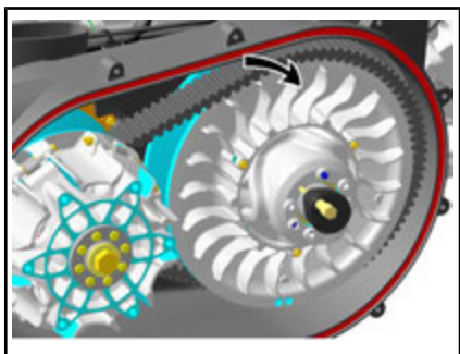
1. Partie la plus basse des pignons alignée avec la surface externe de la courroie d'entraînement
