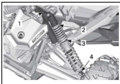
TÍPICO – MODELOS MAVERICK X3 MAX X dsDS E X rsRS – SUSPENSÃO DIANTEIRA
