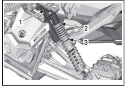
TÍPICO – MODELOS MAVERICK X3 MAX – SUSPENSÃO DIANTEIRA
