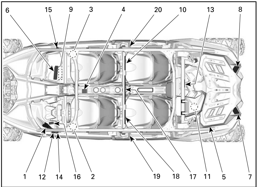
PEÇAS REMOVIDAS PARA MELHOR VISUALIZAÇÃO
