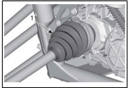
TRASEIRA DO VEÍCULO (COMPONENTES REMOVIDOS PARA MELHOR VISUALIZAÇÃO)
