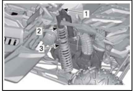
TÍPICO – MODELOS MAVERICK X3 MAX – SUSPENSÃO TRASEIRA
