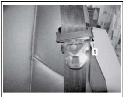
TÍPICO - PEÇAS REMOVIDAS PARA MELHOR VISUALIZAÇÃO
