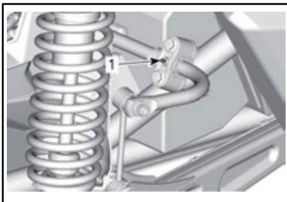
TÍPICO - BARRA ESTABILIZADORA TRASEIRA
