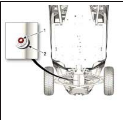
MODÈLES ÉQUIPÉS DU DIFFÉRENTIEL AVANT SMART-LOK
