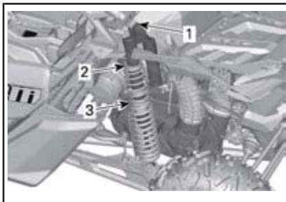
TYPIQUE - MODÈLES MAVERICK X3 MAX - SUSPENSION ARRIÈRE
