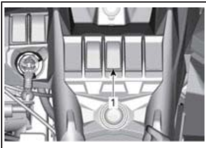
1. Interrupteur du mode du différentiel avant
