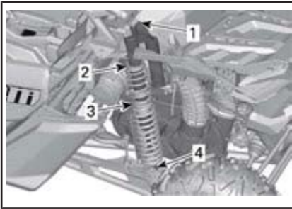
TYPIQUE - MODÈLES MAVERICK X3 MAX X ds DS - SUSPENSION ARRIÈRE
