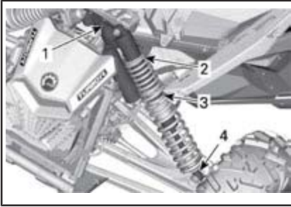
TYPIQUE - MODÈLES MAVERICK X3 MAX X ds DS ET X rs RS - SUSPENSION AVANT
