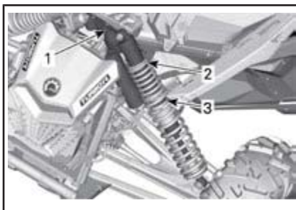
TYPIQUE - MODÈLES MAVERICK X3 MAX - SUSPENSION AVANT
