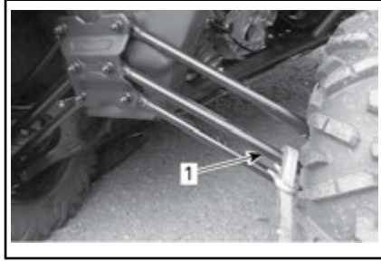
1. 后部中央悬架臂
